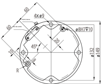
Schéma du socle FR5
