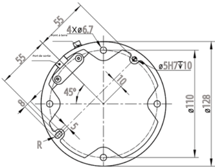
Schéma du socle FR3
