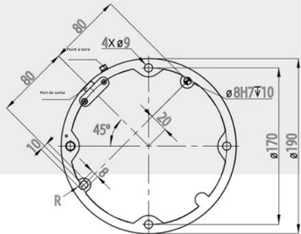
Schéma du socle FR10
